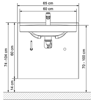
CADRE MANUEL GAUCHE STANDARDLINE AVEC LAVABO WBR-200
